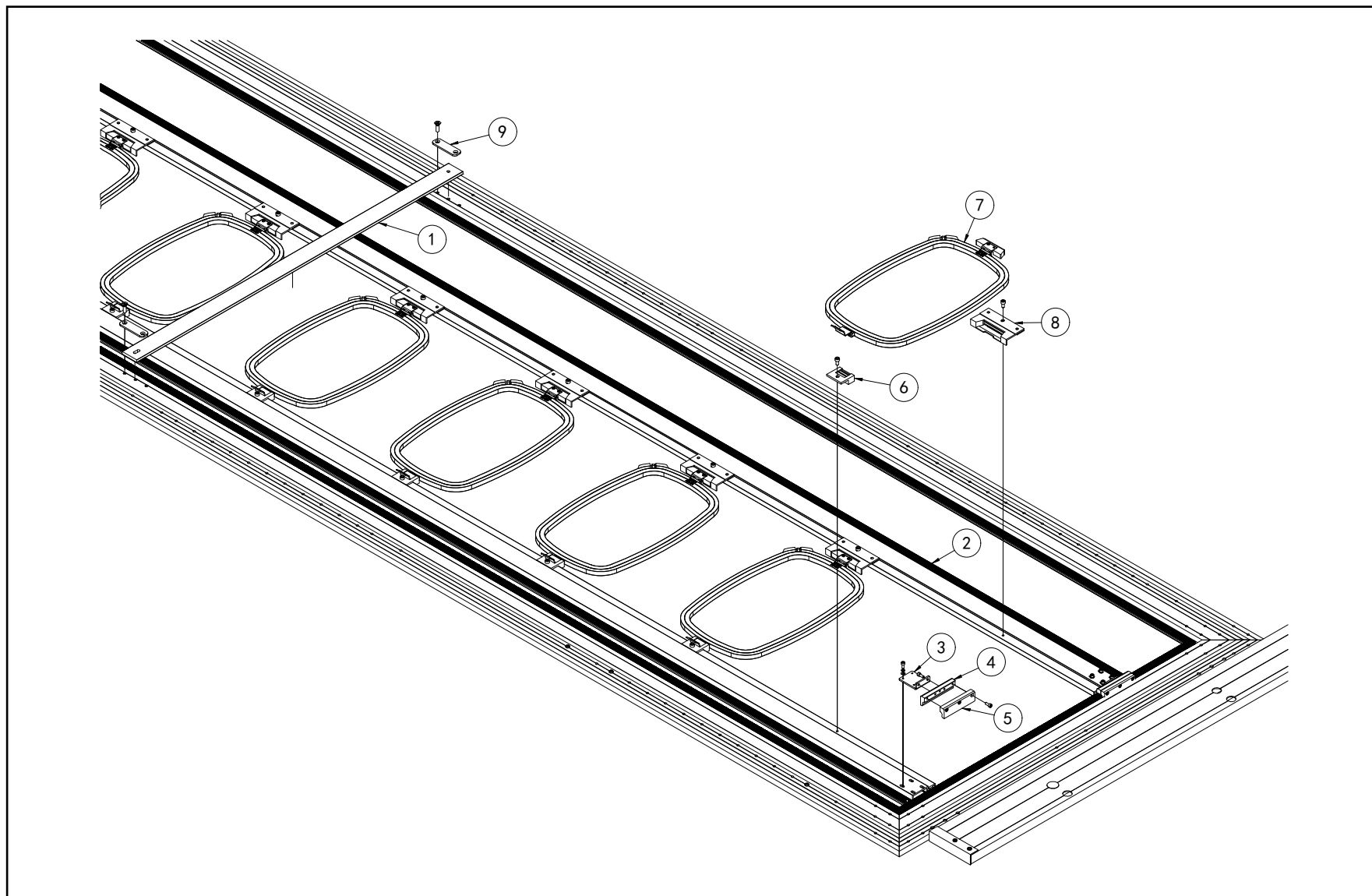
绣框选配部分图
