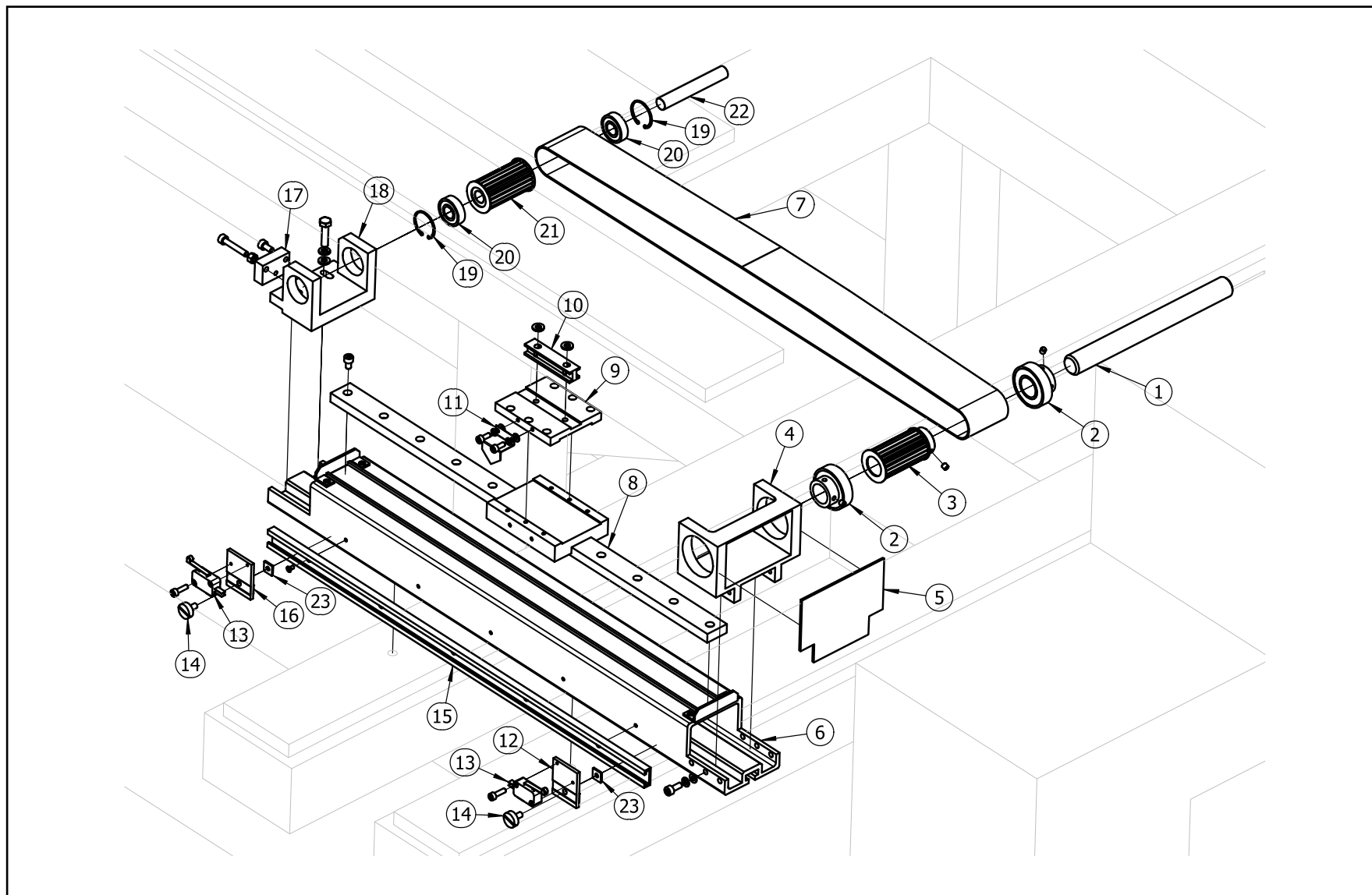
XY轴驱动座部分图
