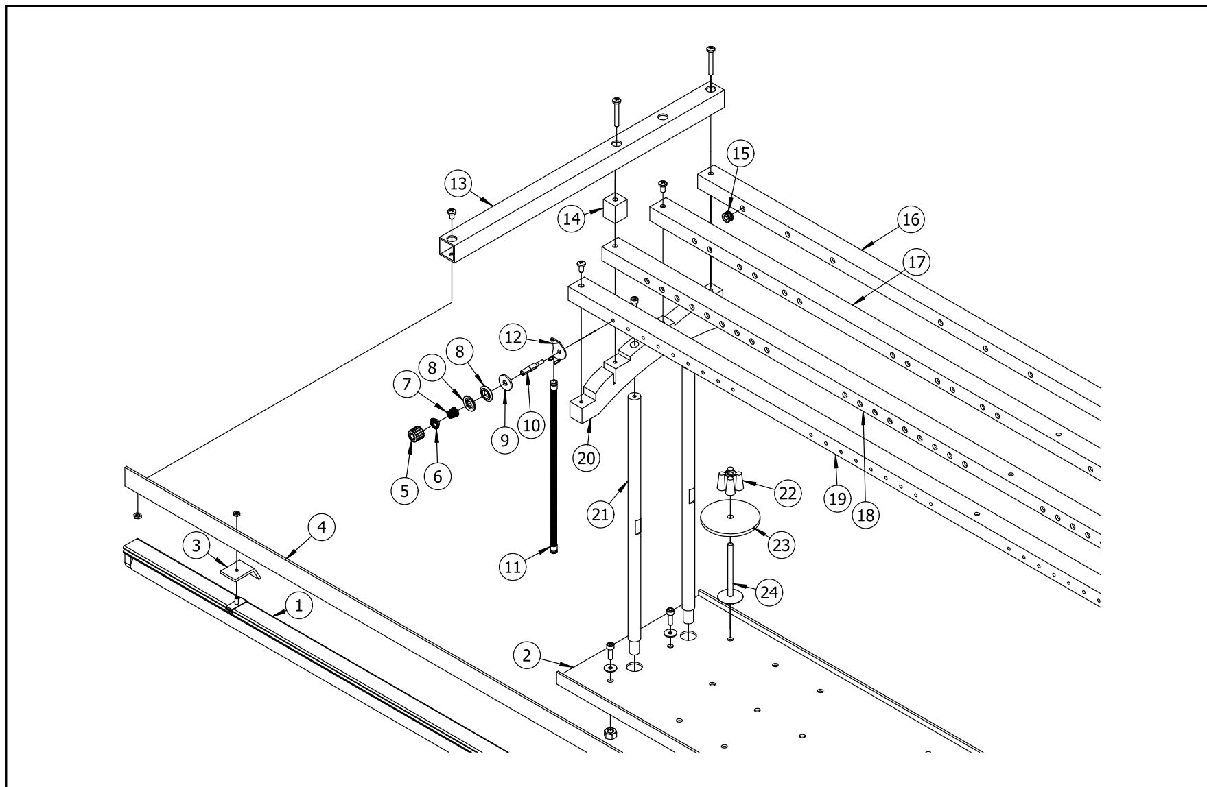
线架部分图
