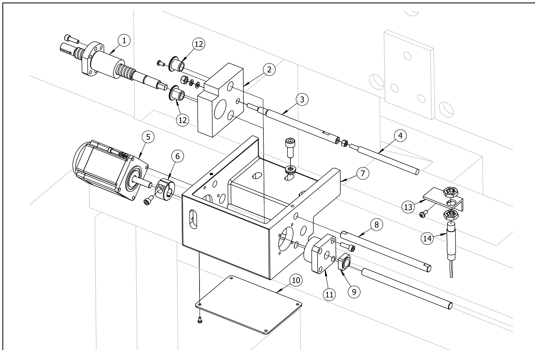
丝杆剪线箱部分图
