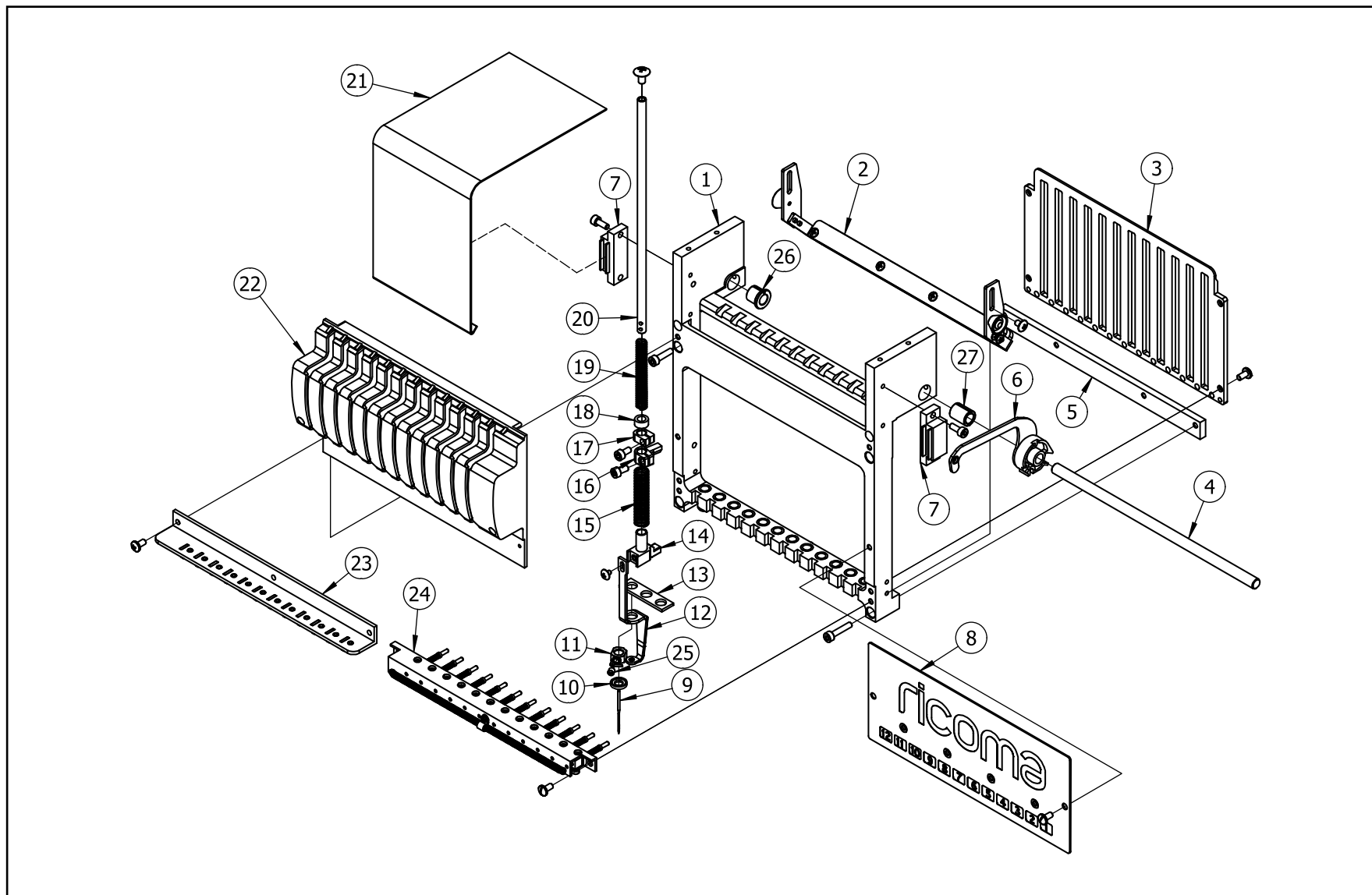
针杆架部分图
