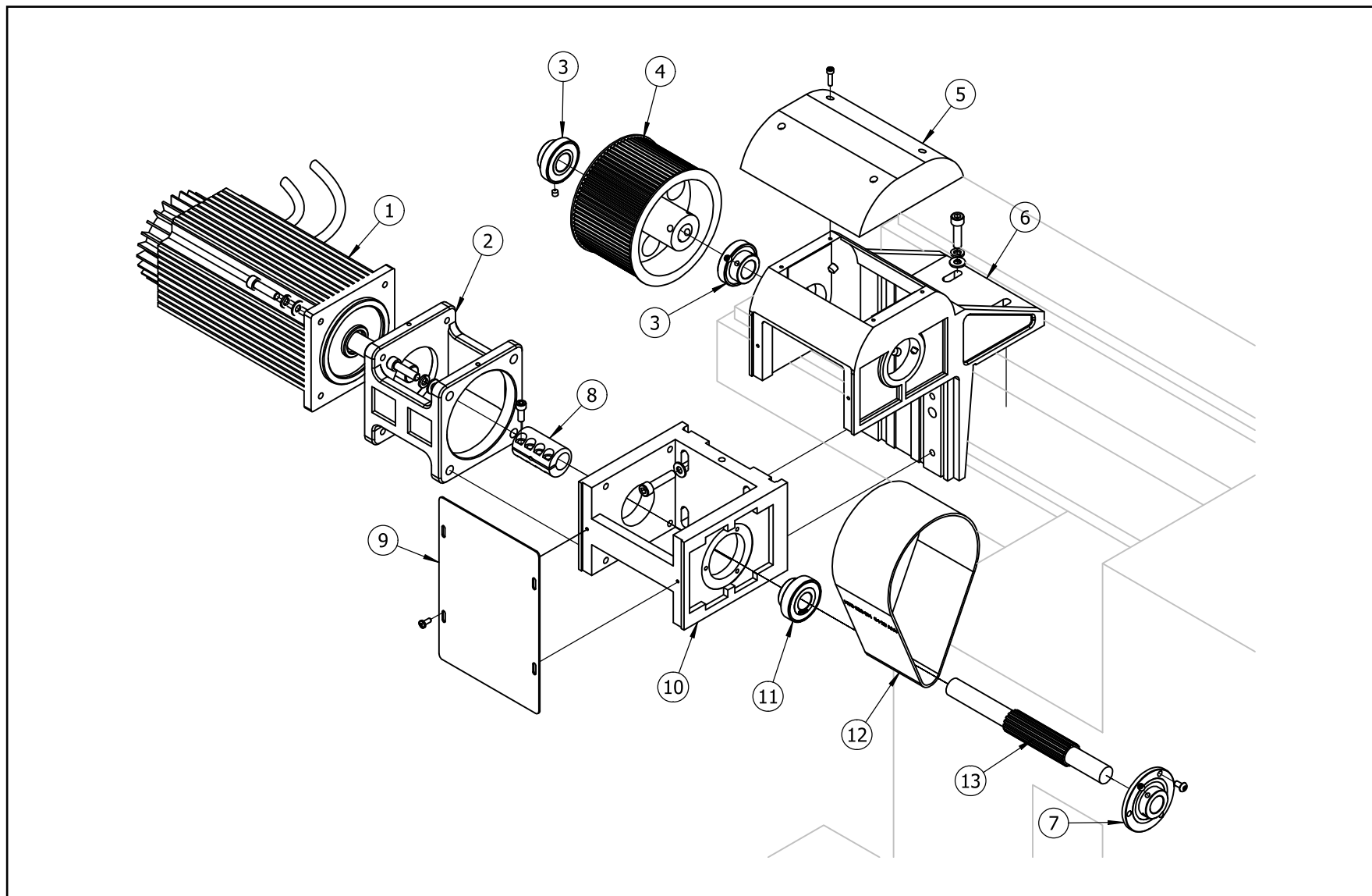
XY伺服传动箱部分图二
