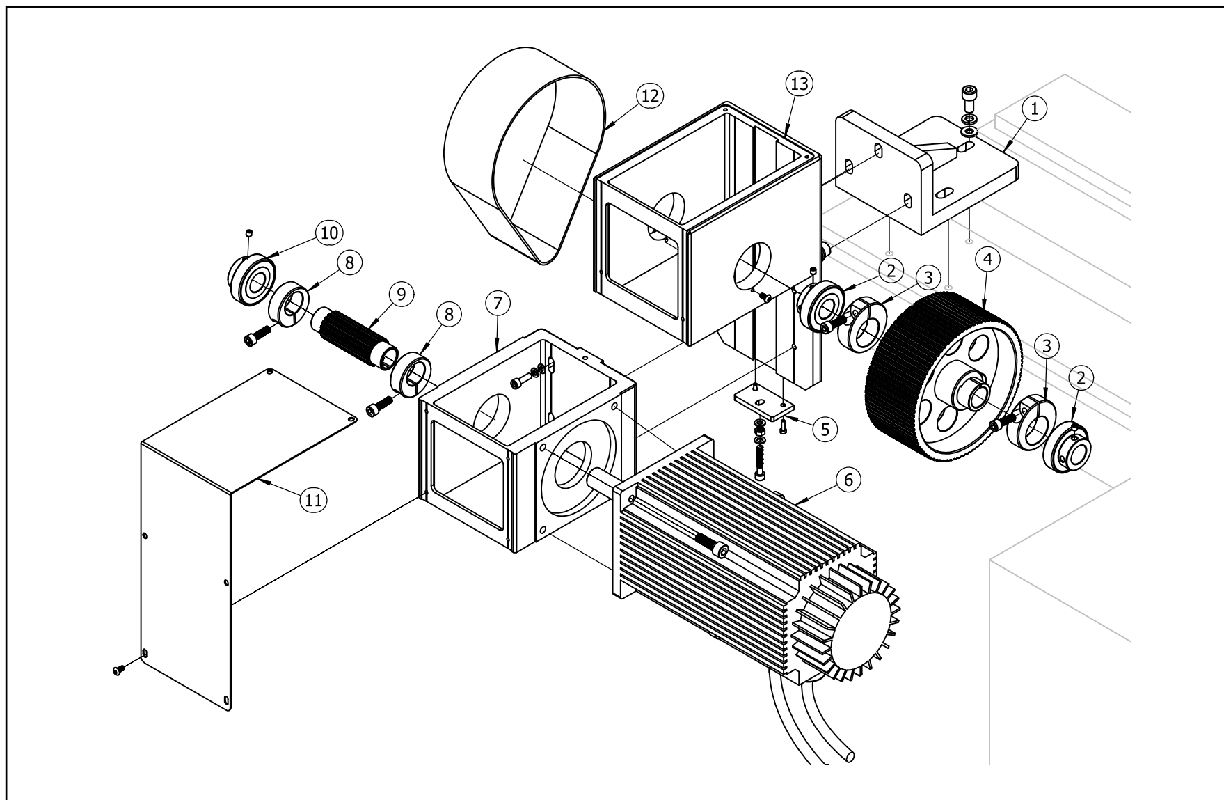
XY伺服传动箱部分图一
