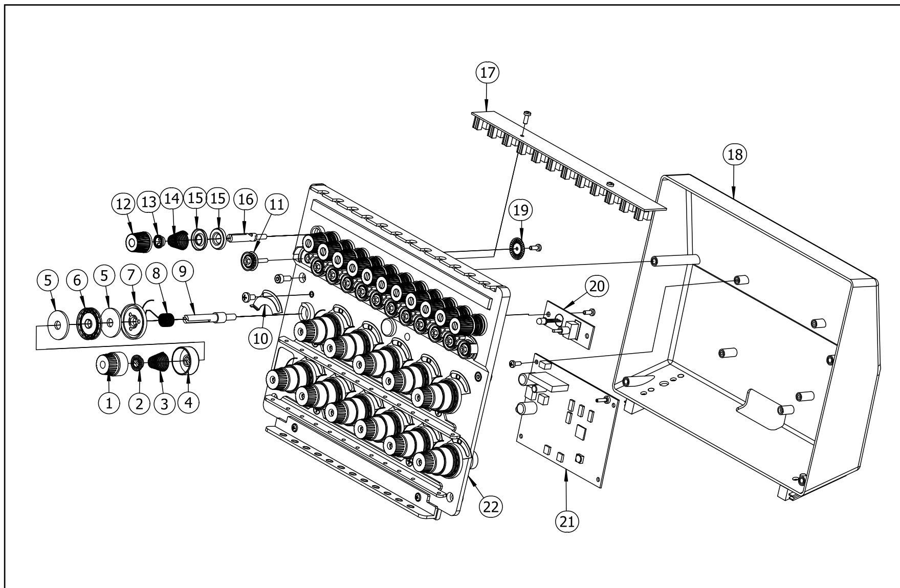
轮+簧夹线器部分图
