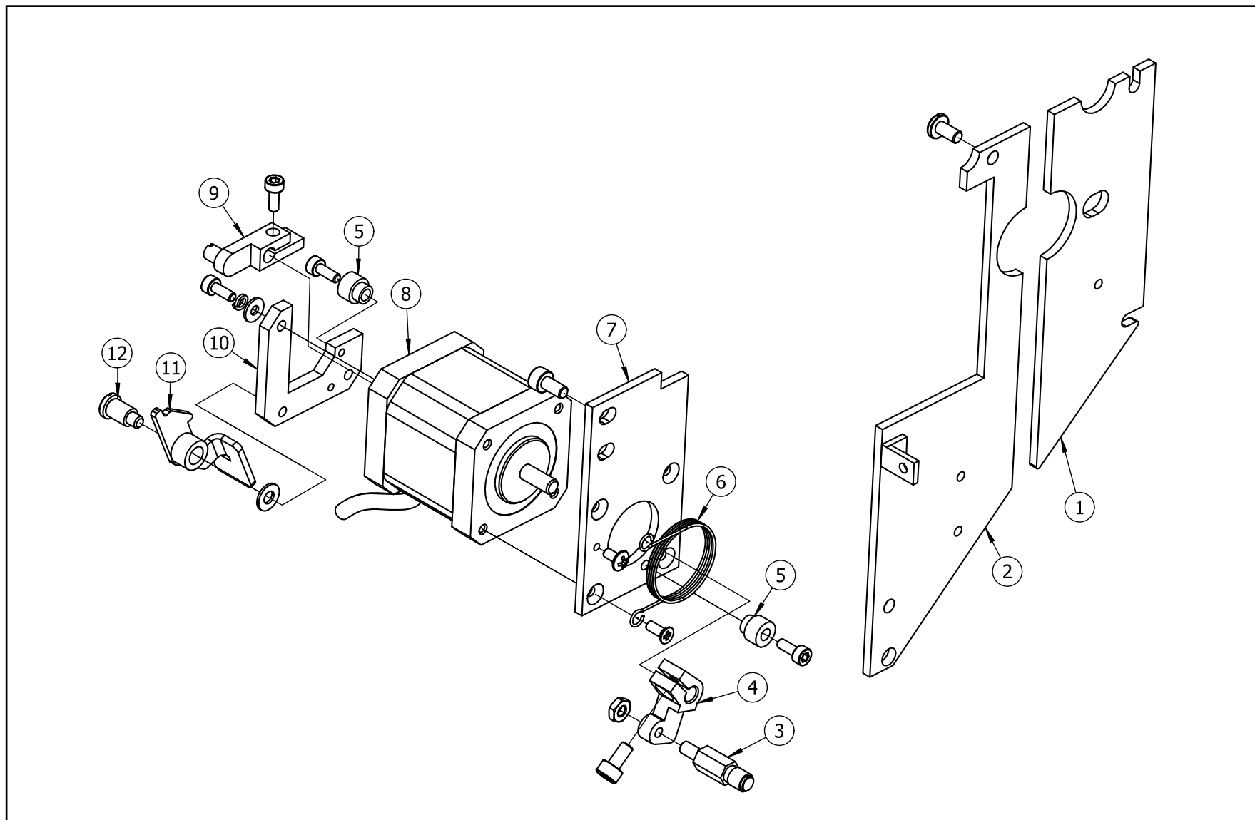
跳跃电机部分图
