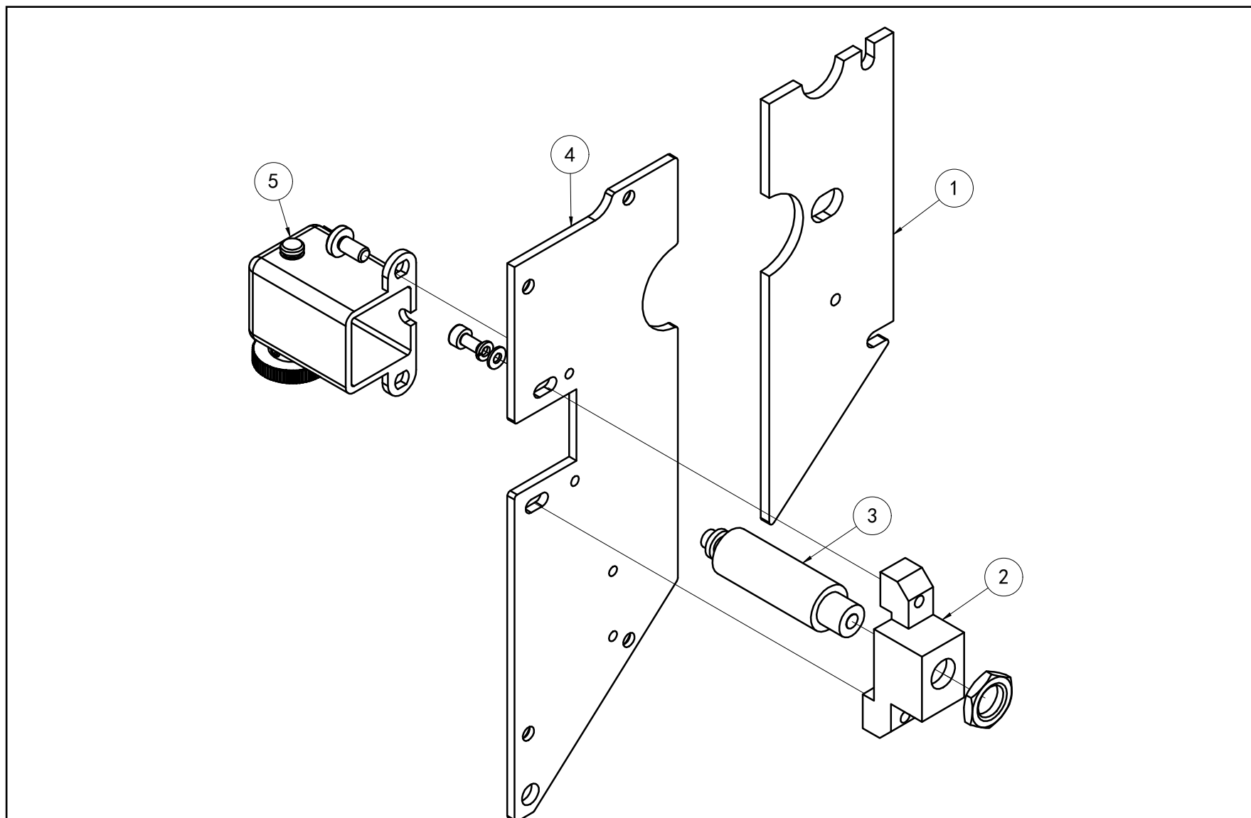
跳跃电磁铁部分图
