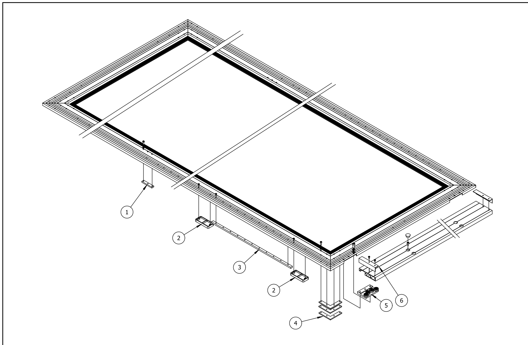
绣框部分图
