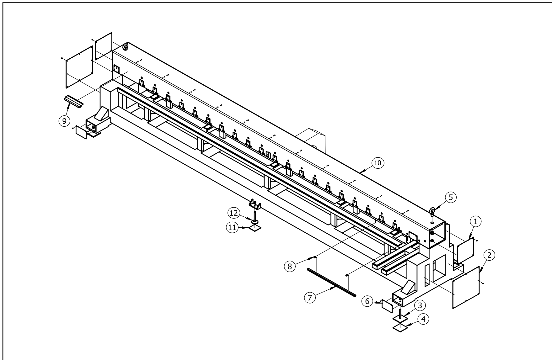
机架部分图
