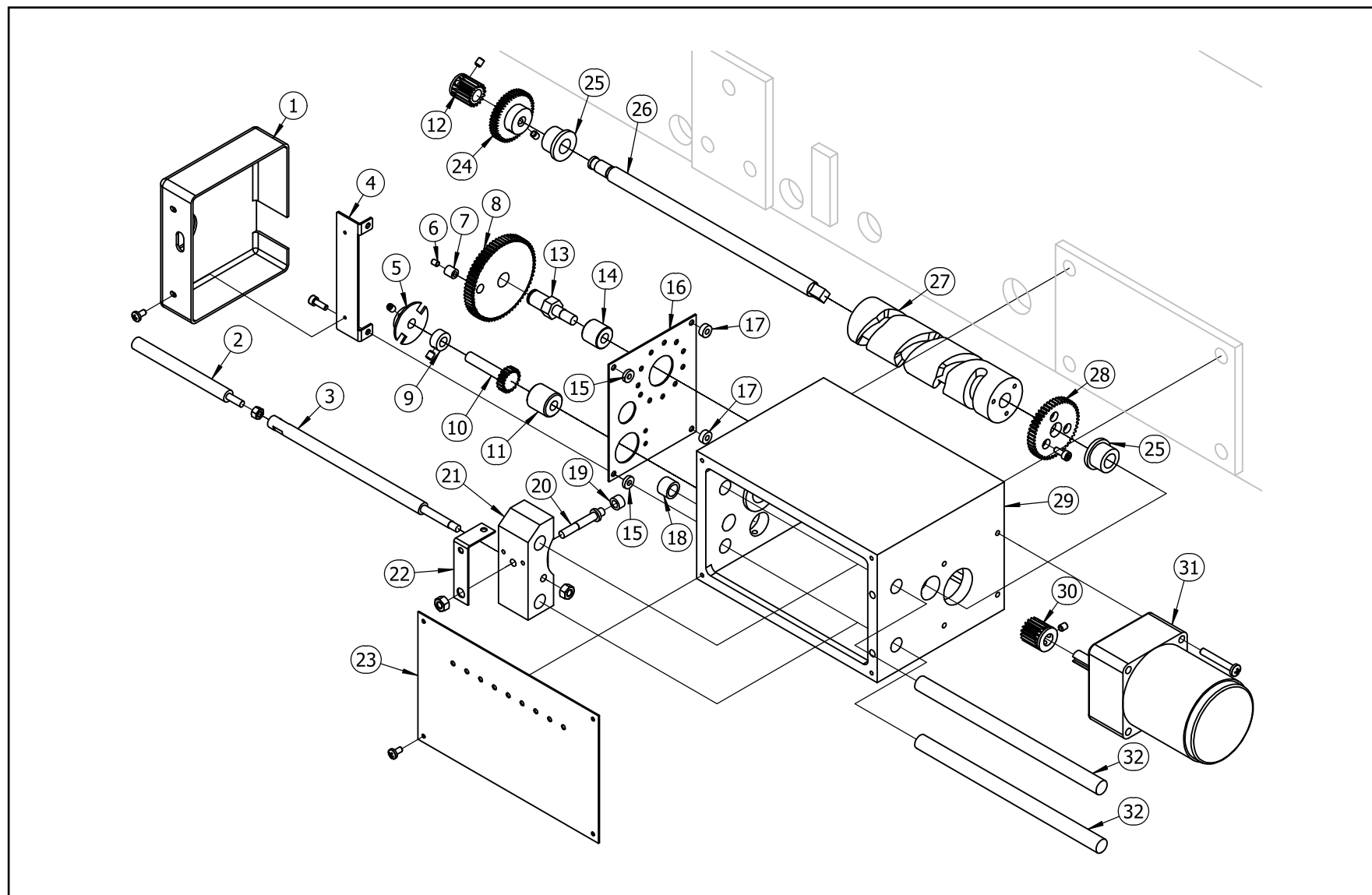
交流换色箱（6、9针）部分图
