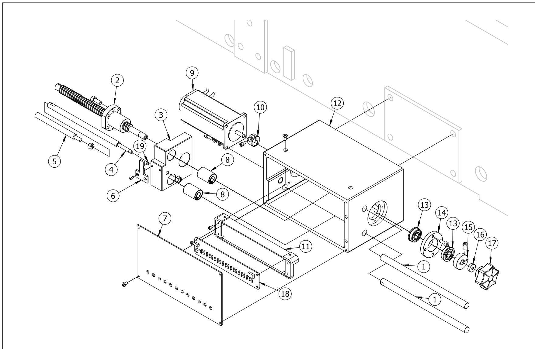
丝杆换色箱部分图
