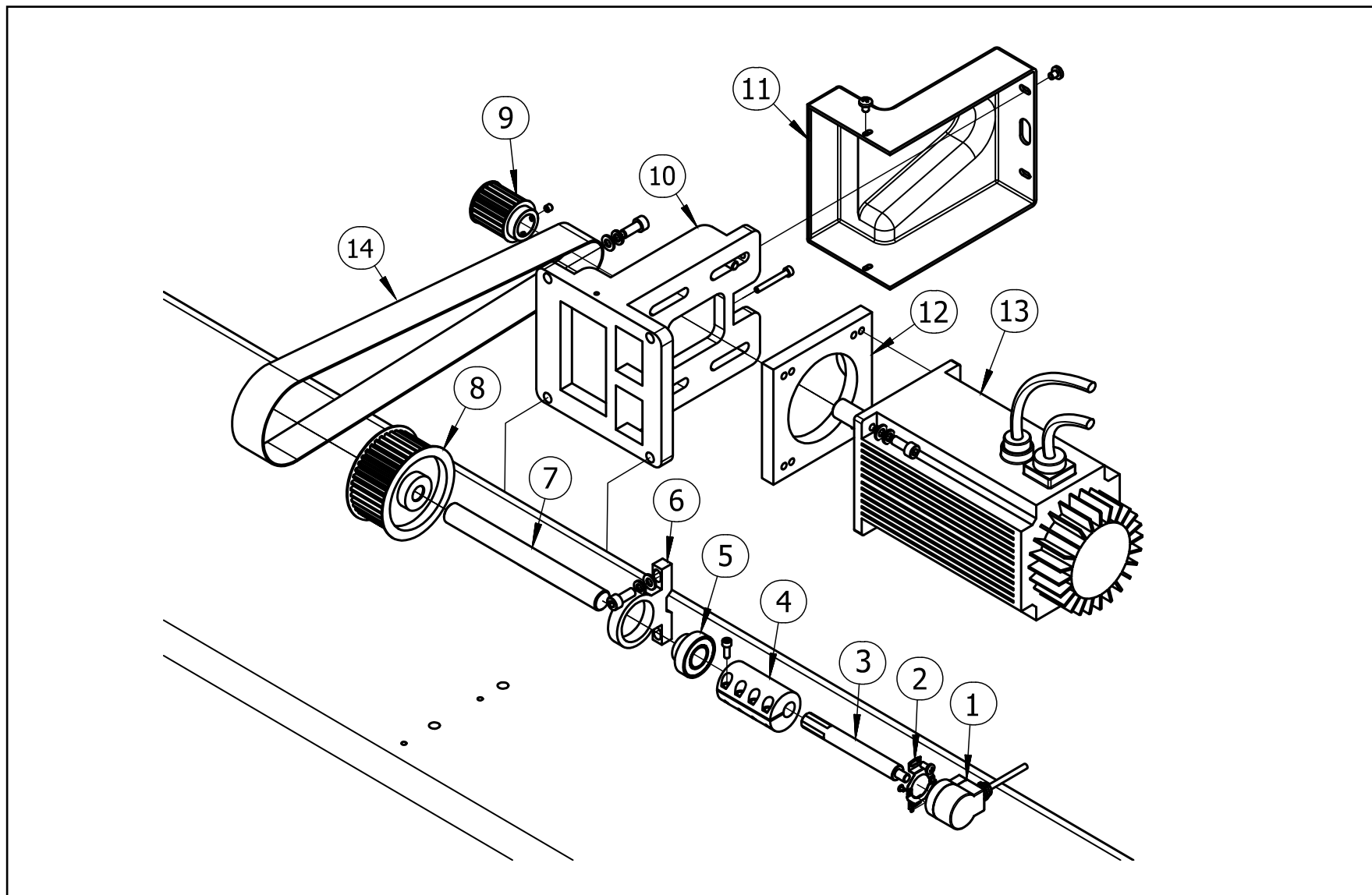
主轴电机传动部分图
