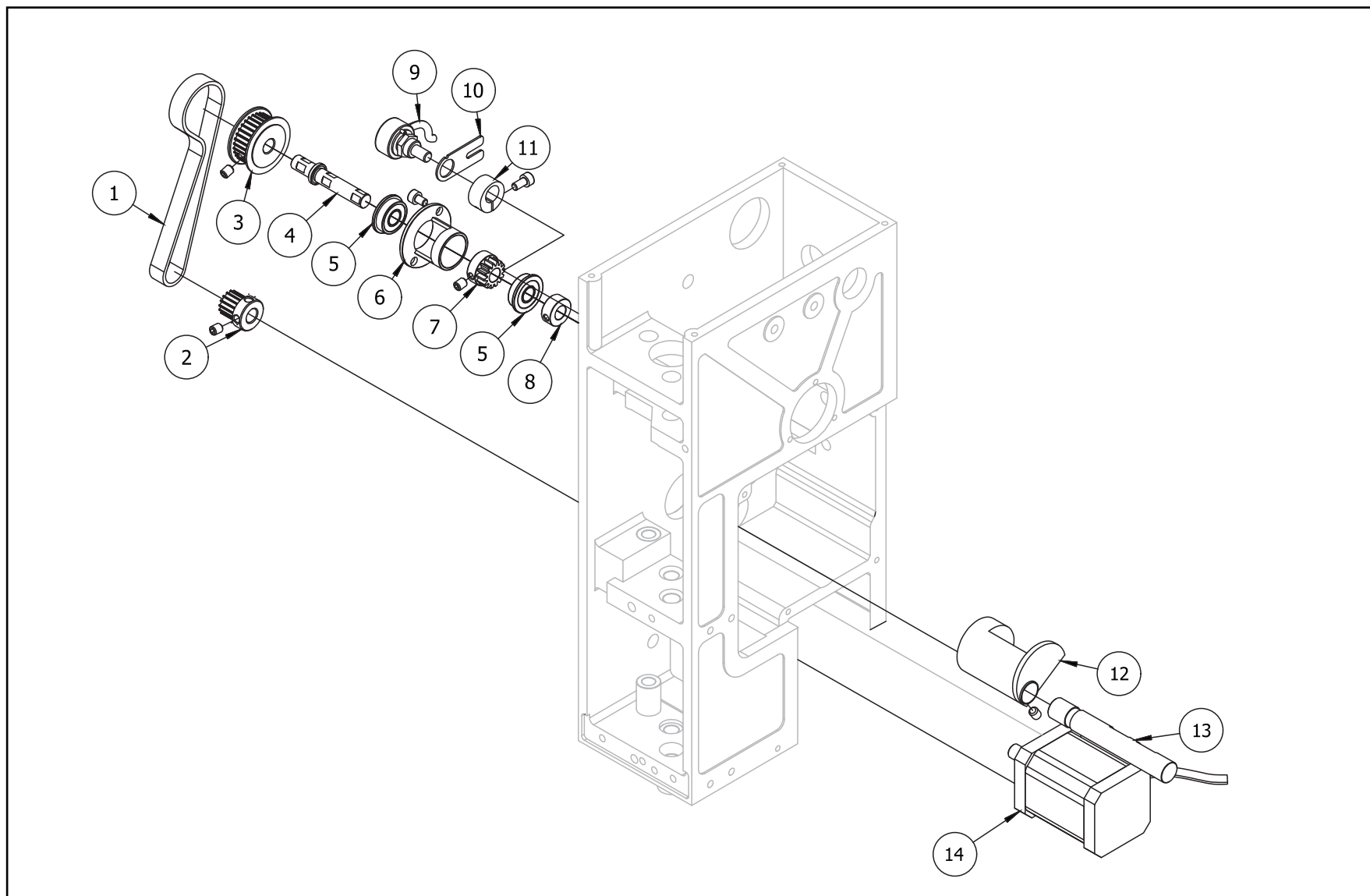
高速毛巾机头部分图三
