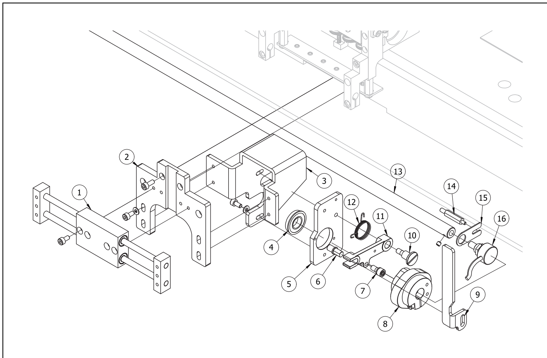
毛巾松线部分图二
