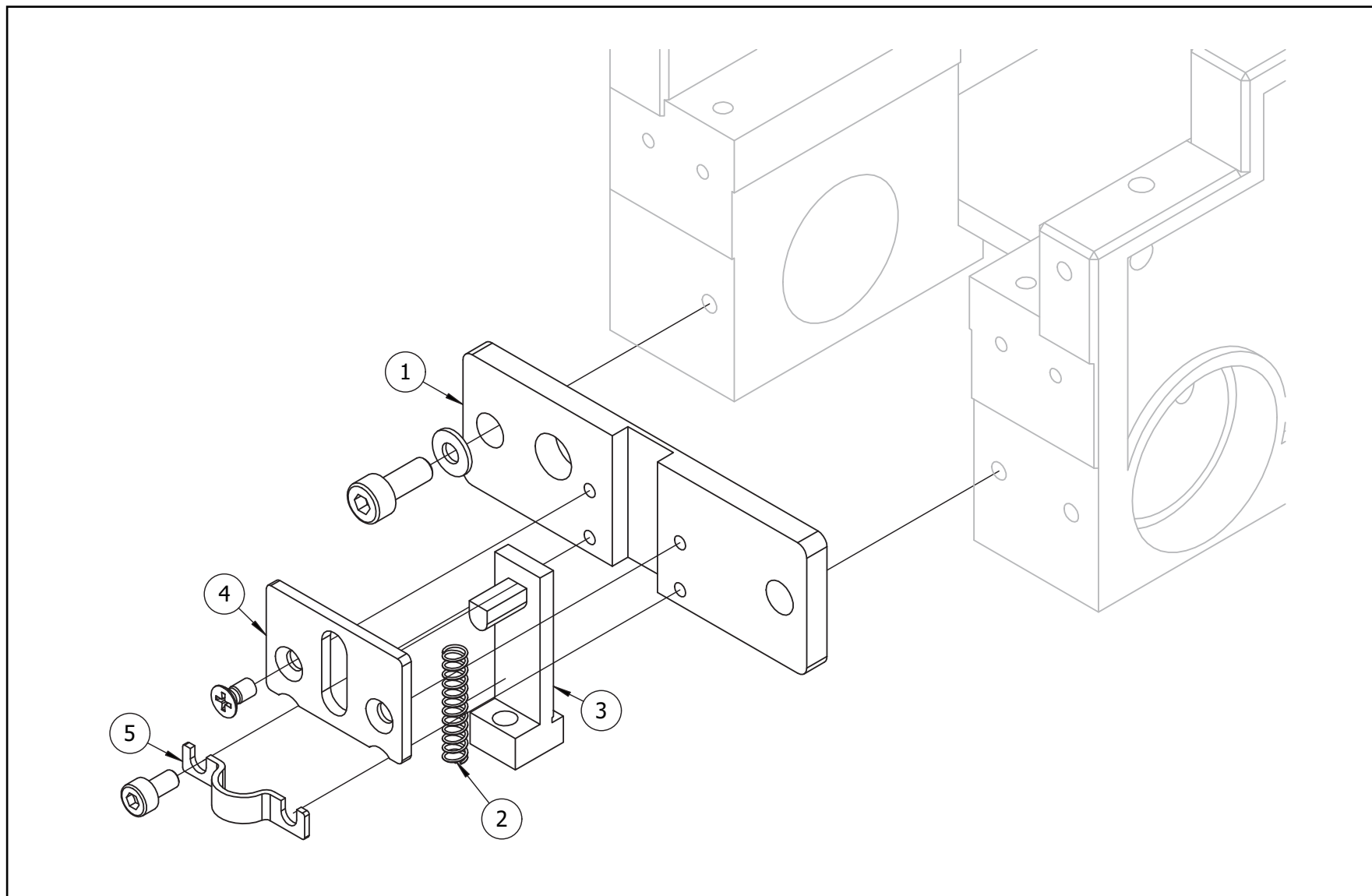
毛巾松线部分图一
