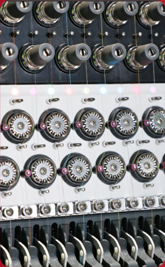
磁编断检 及时发现问题隐患, 有效防止意外停机, 确保刺绣流程连续稳定
